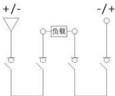
C 型接线方式
